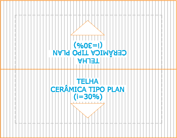
PLANTA DE COBERTURA ESC.: 1:50
